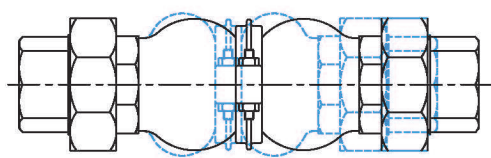
軸向壓縮
