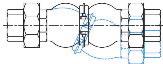
橫向變位
